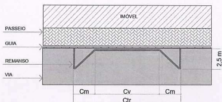
MODELO DE REMANSO S/ ESCALA
