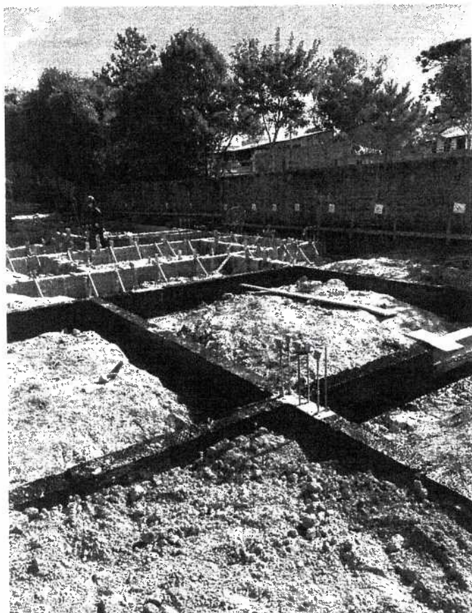
Figura 2 - UBS Silvio Skraba - Estrutura - Vigas de Baldrame
