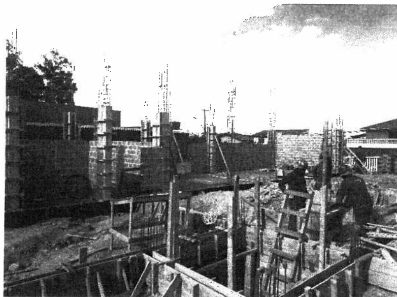
Figura 1 - UBS Silvio Skraba - Alvenaria de elevação
